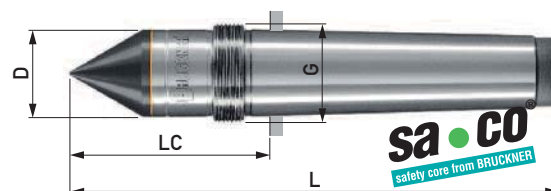
Form GV Spitze Vollhartmetall mit Sicherheitskern sa•co ®
