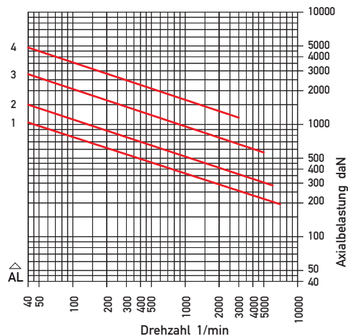
Axial – Typ LKS/LKSG
