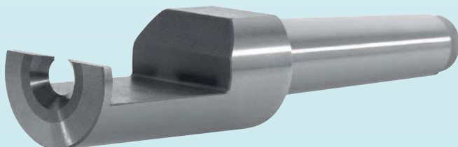
offene Zentrierbohrung
