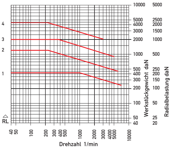
Radial – Typ LKS/LKSG
