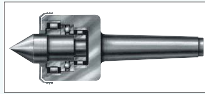
Rotierende Hochleistungsspitze für die Schwerbearbeitung, mit 2 Rollenlagern 1936
