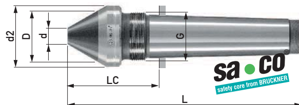
Form GZ großer Hartmetalleinsatz mit Sicherheitskern sa•co ®
