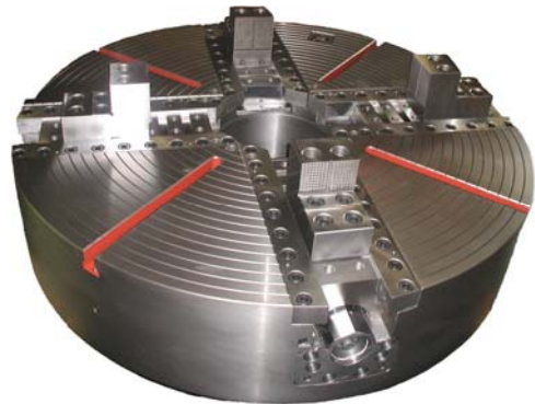
Planscheibe Drm. 1800 mm mit Kraft- spannspindeln Spannkraft 30 To/Backe
