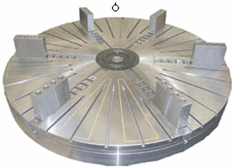
6-Backen-Planscheibe Drm. 1500 mm mit Elektropermanent Magnetsegmente
