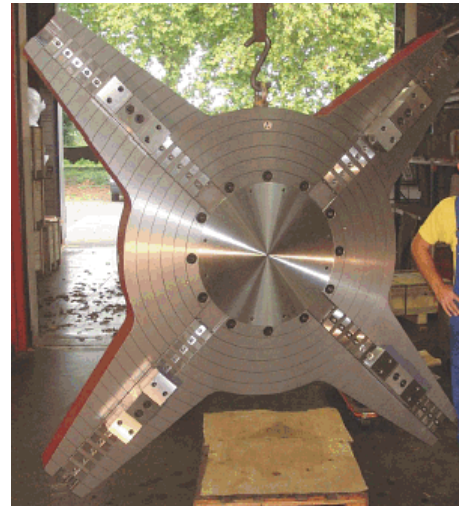
Wescott 4-Backen- Sonderdrehfutter
