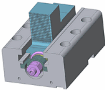
Spannklauenkasten mit Kraftspannspindel Spannkraft 20 to/Backe
