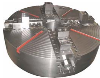
Planscheibe D 1800 mit Kraftspann- spindeln Spannkraft 30 to/Backe
