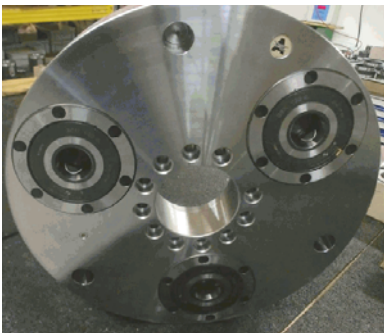
Integrierte Nullpunkt-Spannsysteme sekundenschnelle Positionierung im \mu -Bereich
