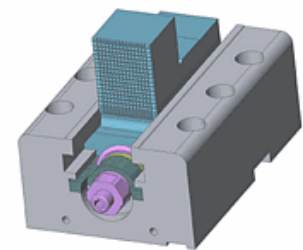
Spannklauekasten mit Kraft- spannspindel 20 to/Backe
