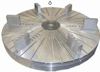
6-Backen-Planscheibe D 1500 mm mit Elektropermanent-Magnetsegmenten
