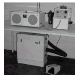
FG 1 Restauo Arbeitsplatz mit Arbeitskabinen und Entstauber FG 1 Restauo work station with work cabin and dust absorber FG 1 Restauo lieu de travail avec cabine de travail et dépoussiéreur
