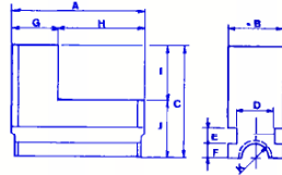
Mors durs reversibles Hardened reversible jaws Gehärtete Umkehrbacken
