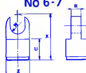
Support de vis Nut Haltebolzen
